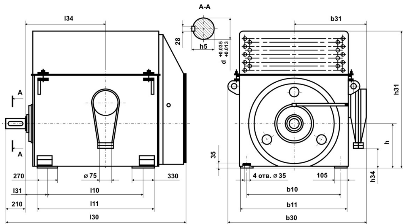
Рис. 2 – электродвигатель ДАЗО4
